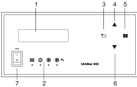
Rys.1 Opis panelu przedniego regulatora
